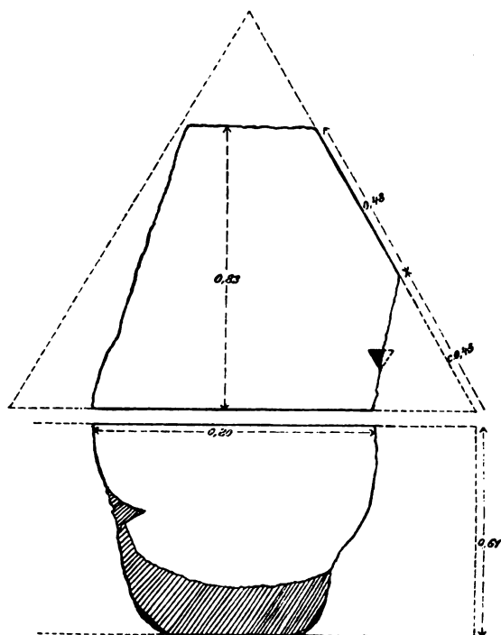
fig. V (1 : 20).
